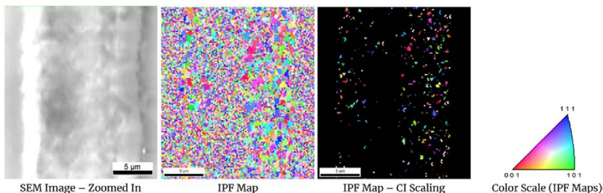
Obr.: SEM a EBSD snímky femtosekundovej laserovej modifikácie povrchu YAG skla. Confidence Index (CI) zobrazený v odtieňoch sivej na elimináciu amorfného skleného pozadia. EBSD = elektrónová spätnorozptylová difrakcia.
