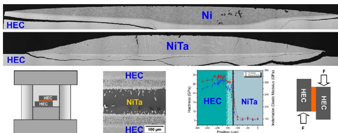
Fig. 1: Grafický abstrakt znázorňujúci zmáčavosť Ni a NiTa na povrchu vysokoentropických karbidov (HEC), schematická ilustrácia procesu spájania a odpovedajúca mikroštruktúra spoja s jeho mechanickými vlastnosťami.
