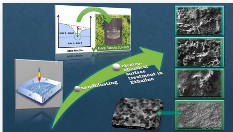
Obr. 1. Morfológie povrchu 3D tlačenej substrátov z titárovej zliatiny po pieskovaní a elektroleštení v hlboko eutektickom rozpúšťadle.
