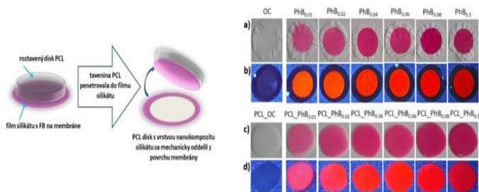
Obr. 1. Schéma prípravy nanokompozitu na povrchu PCL fúziou vrstvy silikátu s taveninou polyméru (hore). Fotografie vrstiev silikátu na membránach (a,b) a ich kompozitov s PCL (c,d) získaných na svetle (a,c) a v tme pod UV lampou (b,d). Čísla v symboloch vzoriek vyjadrujú množstvo PhB ako pomer n_{\text{PhB}} / m_{\text{silikát}} v \text{mmol g}^{-1} .
