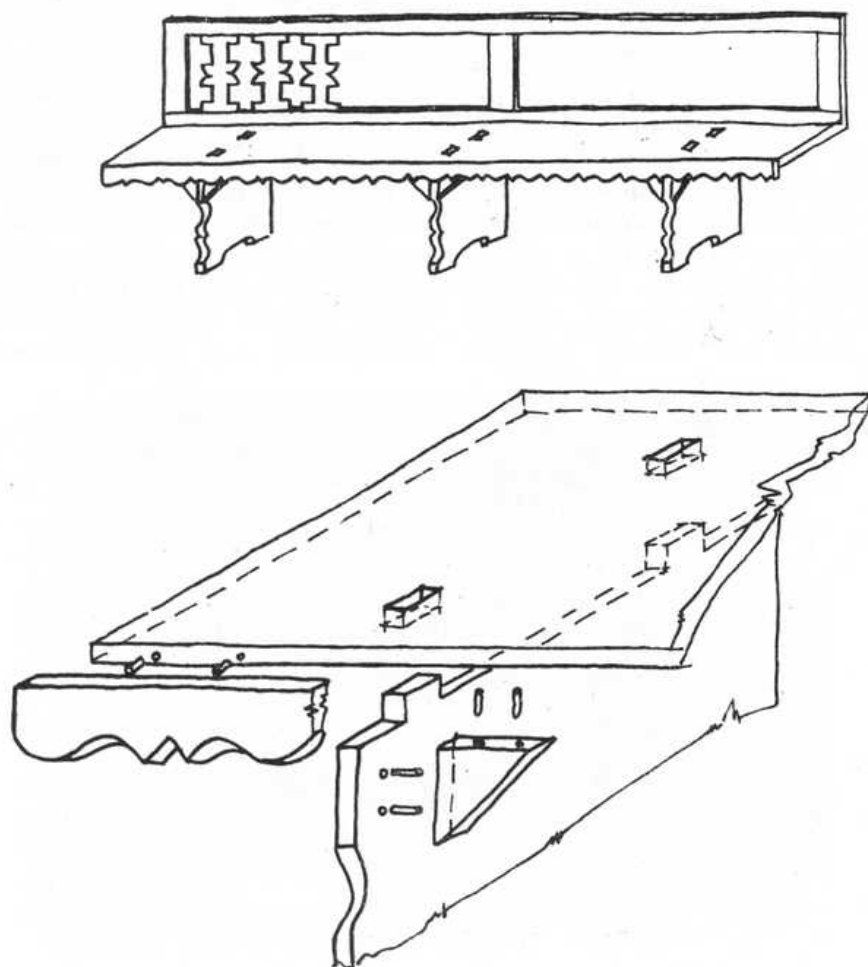
Obr. 12. Lavica do kúta s doskovými nohami; kresba konštrukcie, Starý Tekov.
