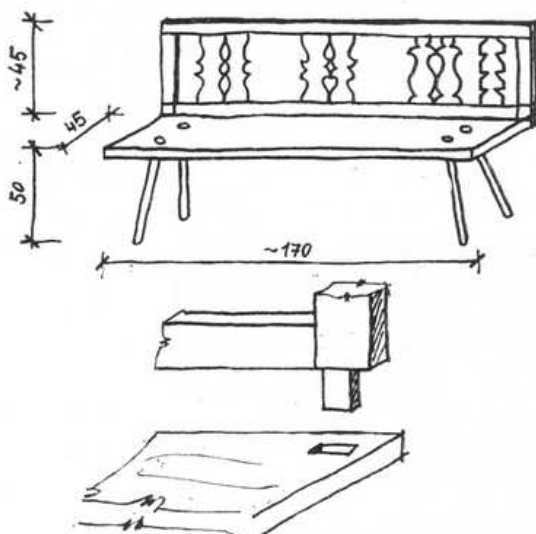
Obr. 8. Lavička s operadlom; kresba spojov jednotlivých častí lavice.
