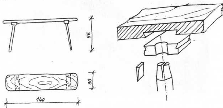
Obr. 7. Kresba konštrukcie stola.
