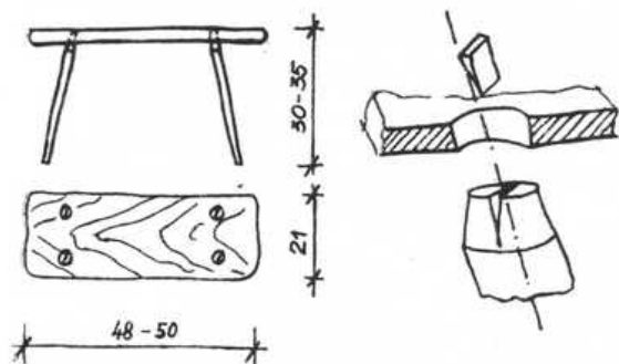
Obr. 18. Stolec na sedenie, a) sedacia časť, b) detail vsadenia nohy s evikom, Starý Tekov.
