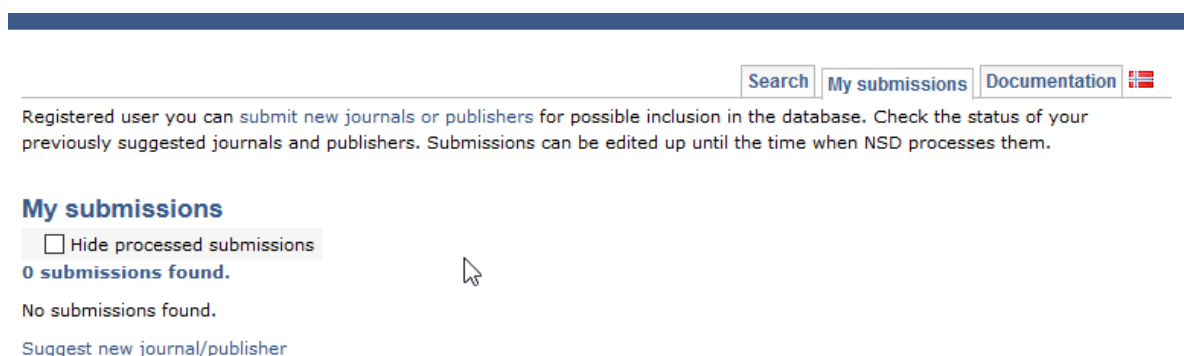
Obrázok 4 My submissions
