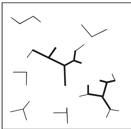
Obr. 1. Štruktúra prvku krajiny – vrstvy
