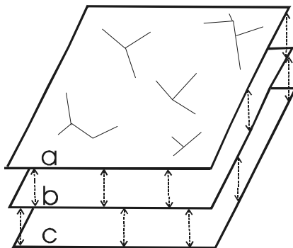
Obr. 2. Štruktúra krajiny – systému
