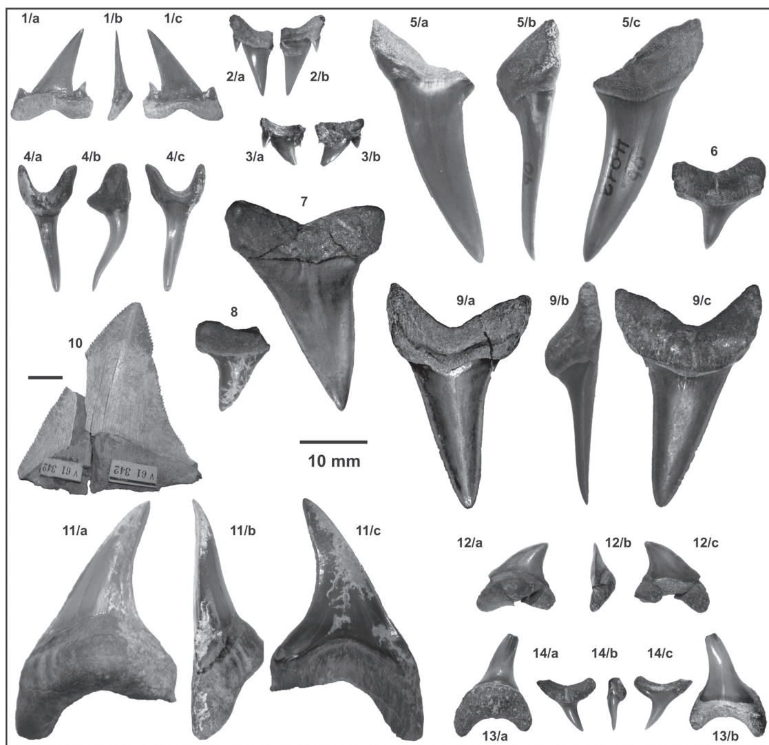
Fig. 5. 1–3 — Carcharoides catticus : 1 — lateral (IT-98), lin (a), mes (b), lab (c); 2 — anterior (IT-98) lin (a), lab (b); 3 — lateral (IT-M16-3) lab (a), lin (b). 4–6 — Isurus desori : 4 — second anterior (IT-III-134) from juvenile specimens, lin (a), mes (b) and lab (c); 5 — second anterior from adult specimen (MÁFI-V4813), lab (a), mes (b) and lin (c); 6 — posterior (IT-8). 7–8 — Isurus hastalis : 7 — first lateral (MÁFI-V14928), lab; 8 — posterior (MÁFI-V1616). 9 — Isurus retroflexus : anterior (MÁFI-V14928), lab (a), mes (b), lin (c). 10 — Carcharocles sp: lateral (?) (MTM-V61-342). 11–12 — Parotodus benedeni : 11 — second anterior (MÁFI-V14946) and 12 — posterior (MÁFI-V14940), lin (a), mes (b) lab (c). 13–14 — Alopias exigua : 13 — first lateral (IT-118), lin (a) lab (b); 14 — lateral (IT-87), lin (a), mes (b) lab (c). (The small scale bar (10 mm) for Fig. 7.)
