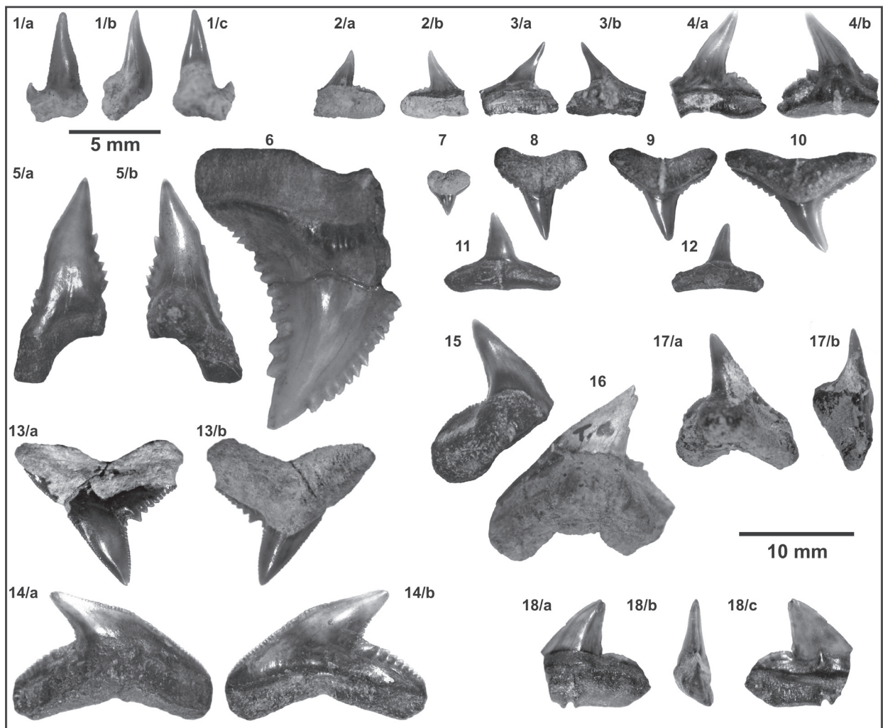
Fig. 6. 1 — ? Scyliorhinus sp.: anteroposterior (IT-M19-8), lab (a), mes (b), lin (c), (scale bar: 5 mm). 2–4 — ? Paragaleus sp.: anterolaterals 2 — lin (a), lab (b) (IT-V-6); 3 — lab (a), lin (b) (IT-II-36); 4 — lab (a), lin (b) (MÁFI-V14906). 5–6 — Hemipristis serra : 5 — first lateral (MÁFI-V14939), lab (a) lin (b); 6 — lateral (MÁFI-V14911), lab. 7–12 — Carcharhinus prisca : 7 — medial (IT-M16-4); 8–9 — anterior (IT-100 and IT-II-70); 10 — lateroposterior (IT-119); 11–12 — anteroposteriors (MÁFI-V1623 and IT-III-62). 13–14 — Galeocерdo aduncus : 13 — medial (IT-III-23), lab (a), lin (b); 14 — anteroposterior (MÁFI-V14905), lin (a), lab (b). 15–17 — Galeocерdo contortus : 15 — anteroposterior (IT-35); 16 — anterolateral (MÁFI-V14905); 17 — symphysial (MÁFI-V14907), lin (a), mes (b). 18 — Sphyrna cf. zygaena : lateral (MÁFI-V14934), lin (a), mes (b), lab (c). (5 mm scale for Fig. 1.)
