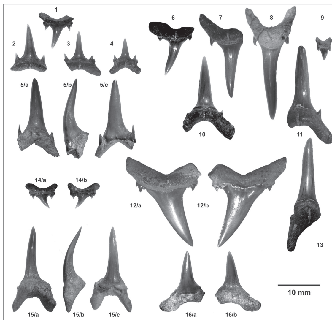
Fig. 4. 1–4 — Odontaspis sp. 1.: 1 — lateral (MÁFI-V14908); 2 — anterior (?) (MÁFI-V14922); 3–4 — laterals (MÁFI-V14908). 5 — Odontaspis sp. 2.: anterior (IT-III-65), lin (a), mes (b), lab (c). 6–11 — Carcharias acutissima : 6 — lateral (MÁFI-V5095); 7 — third anterior (MÁFI-V1621); 8 — first anterior (IT-III-137); 9 — intermediate (IT-108); 10 — lateral (II-133); 11 — first anterior (MTM-V61-322). 12–13 — Carcharias cuspidatus : 12 — lateral (MÁFI-V14937), lin (a), lab (b); 13 — symphysial (MÁFI-V2273&V2275). 14 — Carcharias sp.: lateral (IT-M18-2), lin (a), lab (b). 15–16 — Mitsukurina lineata : 15 — lateral (IT-103), lab (a), lin (b); 16 — anterior (IT-82), lin (a), mes (b), lab (c).
