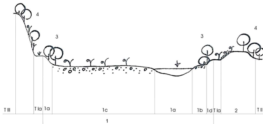
Obr. 5. Pričný rez ripariálnou zónou toku
