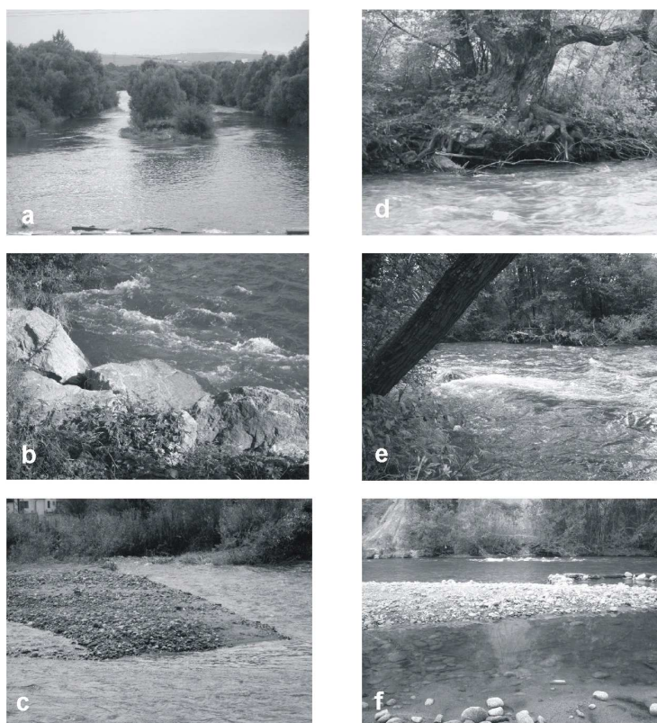
Obr. 6. Príklady hydromorfologickej rôznorodosti Váhu v hornom Liptove
